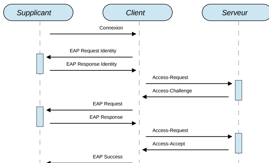
FIGURE 2.2 – Logigramme de connexion à un réseau 802.1X
